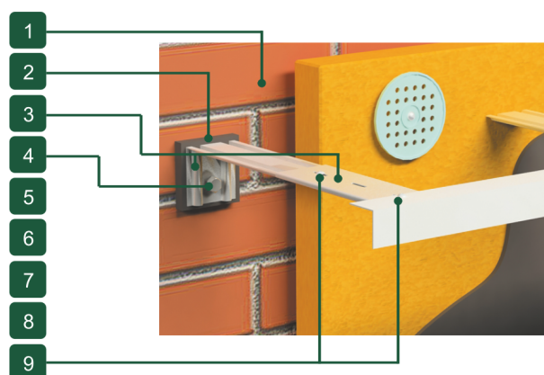
Узел крепления
